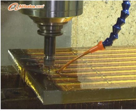
模具压铸
